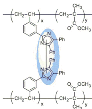
架橋／解架橋性高分子
